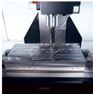
Mynx 6500 Milling
