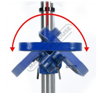
Tilting Table
