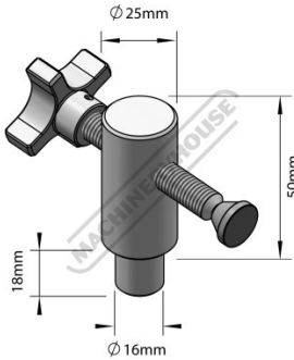
Dimensions
